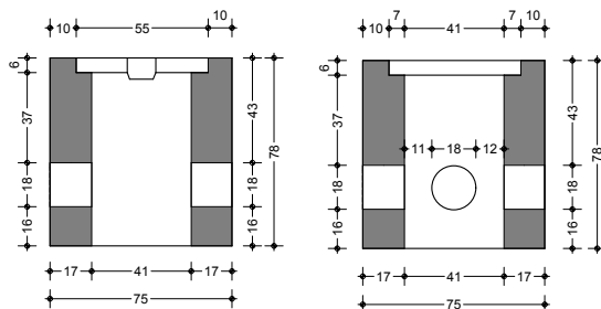
SEZIONE B-B
